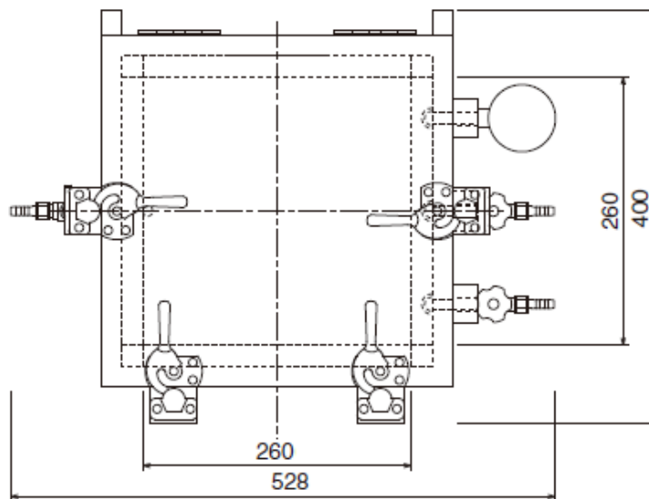
Чертеж UB-D (размеры указаны в мм)
