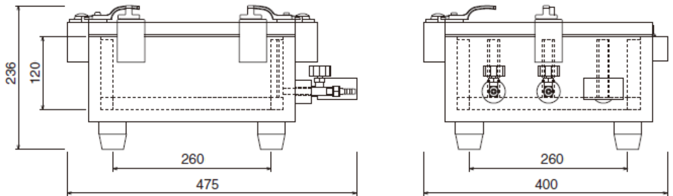
Чертеж UB (размеры указаны в мм)
